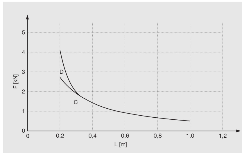
Endefeste WBD 41/45/2,5 D. Belastningsdiagram
