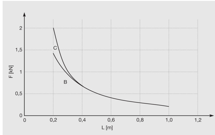
Endefeste WBD 41/52/2,5 D. Belastningsdiagram
