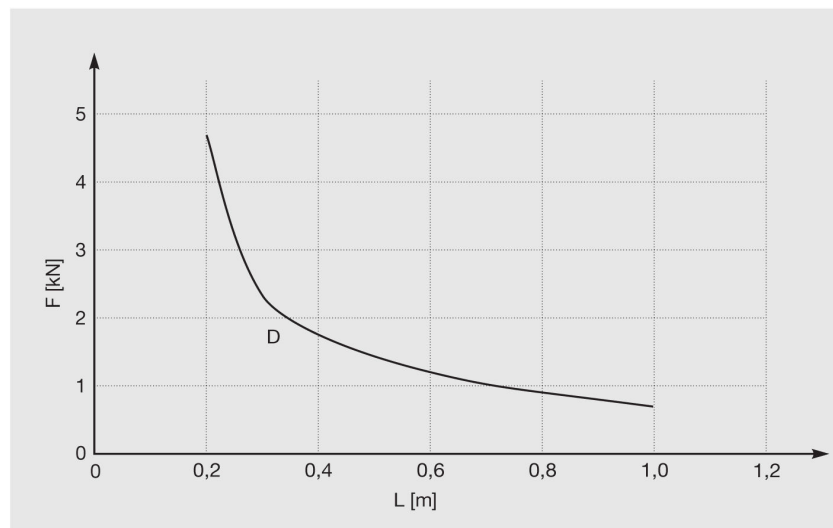
Endefeste WBD 41/52/2,5 D. Belastningsdiagram
