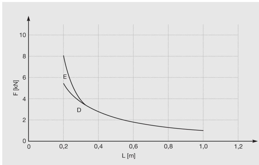
Endefeste WBD 41/62/2,5 D. Belastningsdiagram
